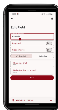
Egyéni mezők
