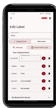
Címke beállítások
